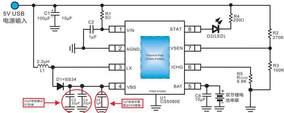
CS5080E充电线路图
